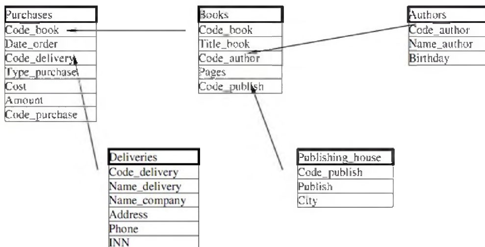
Фрагмент базы данных «Книжное дело»
